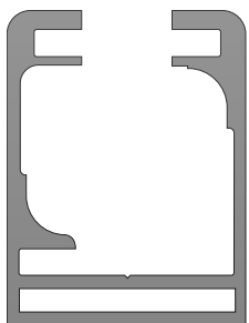
پروفیل کاسا Kasa Profili Main Profile-Bodywork
