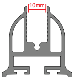
پروفیل بازا (۱۰ میلی) Baza Profili (10mm) Panel Profile (10mm)
