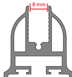
پروفیل بازا (۸ میلی) Baza Profili (8mm) Panel Profile (8mm)
